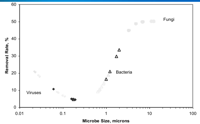
Figura 4: Tassi di rimozione per patogeni nosocomiali disposti in un formato di curva delle prestazioni del filtro MERV 6
